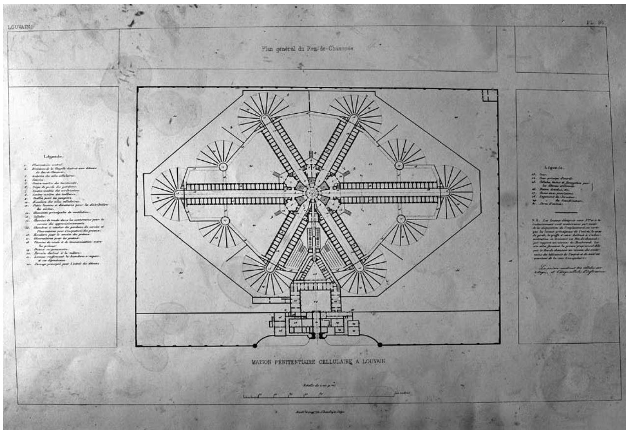
oorspronkelijk grondplan van de Centrale Gevangenis Leuven
